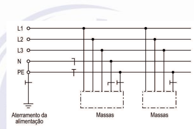
Figura 1 — Esquema TN-S
